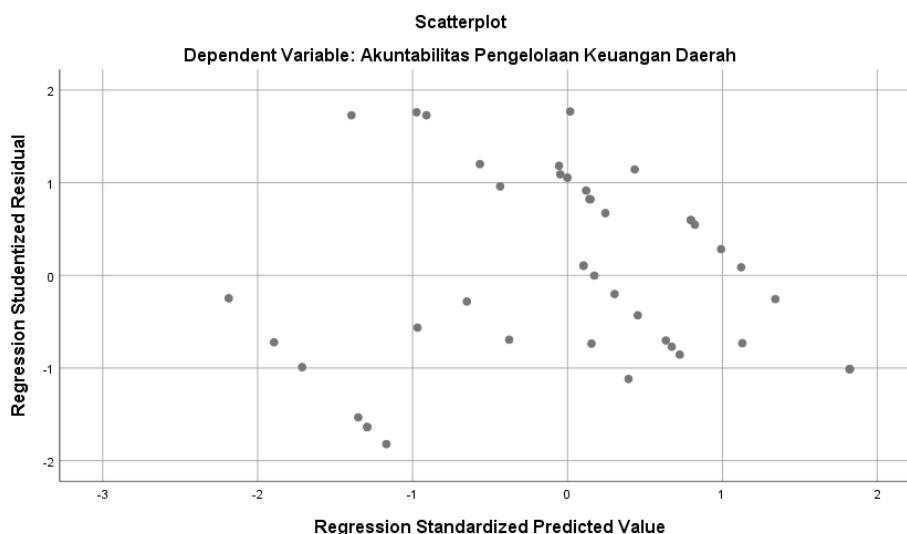
Gambar 1 Grafik Scatterplot
